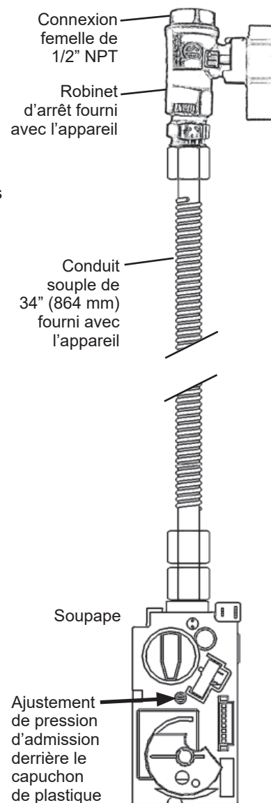
Assemblage de la soupape
